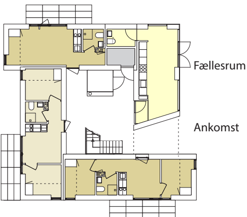
Stueplan
